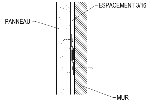
DÉTAIL D'ANCRAGE AU MUR
