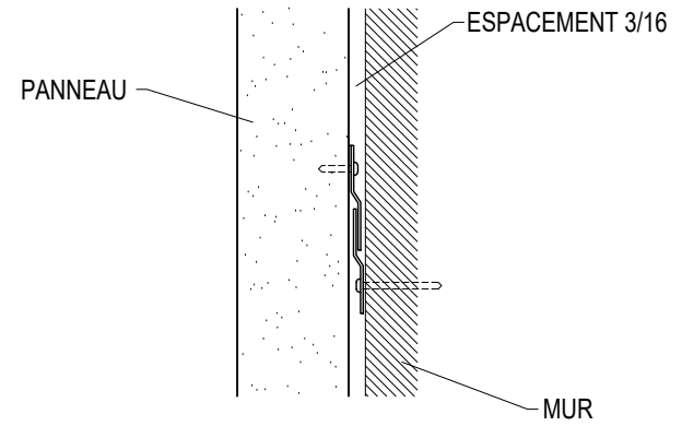
DÉTAIL D'ANCRAGE AU MUR
